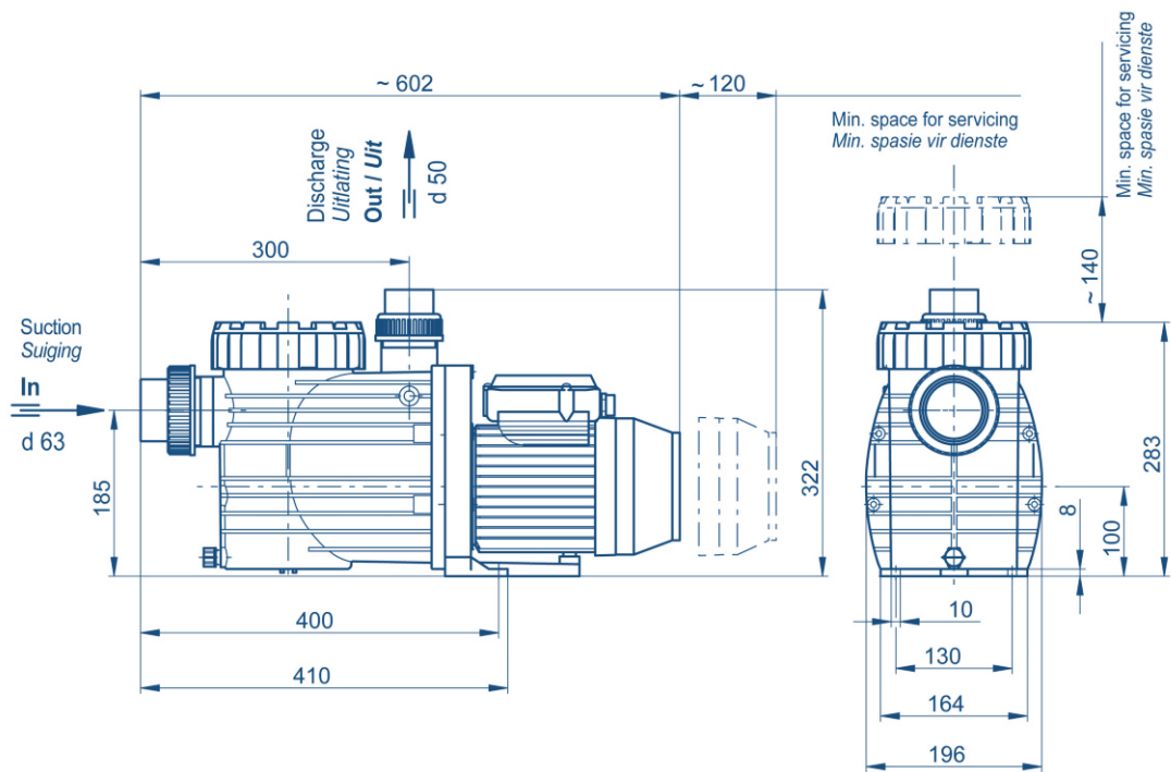
BADU ® Eco Touch dimension table (mm) / BADU ® Eco Touch-afmetingstabel (mm)
